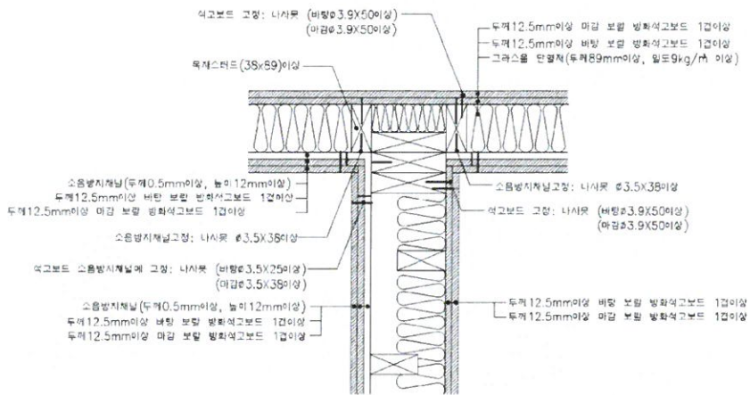
나. “T” 접합상세도
