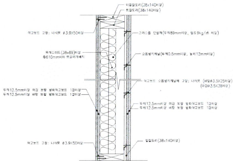
[수평단면 상세도]
