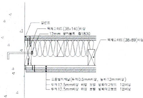
다. 벽 접합상세도
