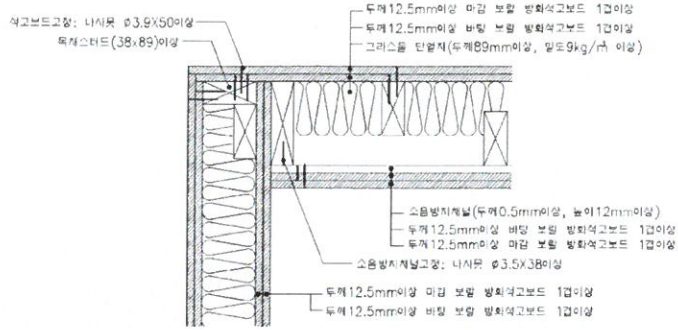
가. “ㄱ” 접합상세도
