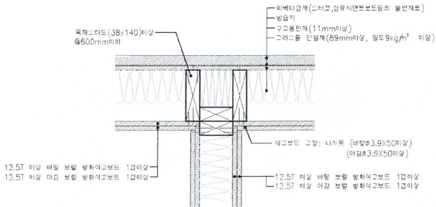
< “T” 접합 상세도 >
