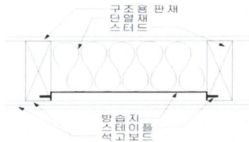
그림 2 단열재의 설치
