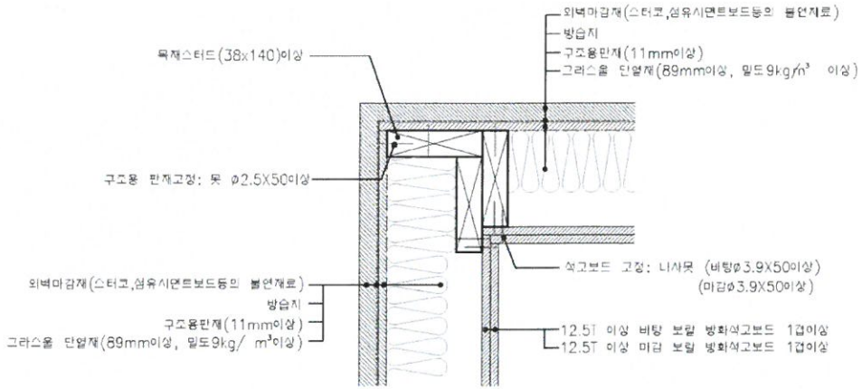
< “G” 접합 상세도 >
