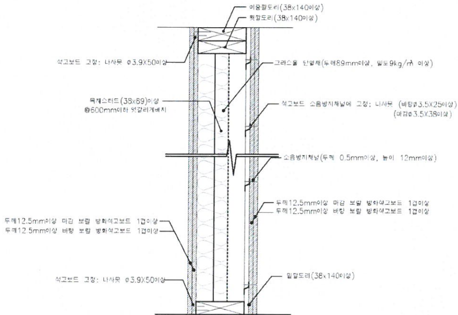
<수직 단면도>
