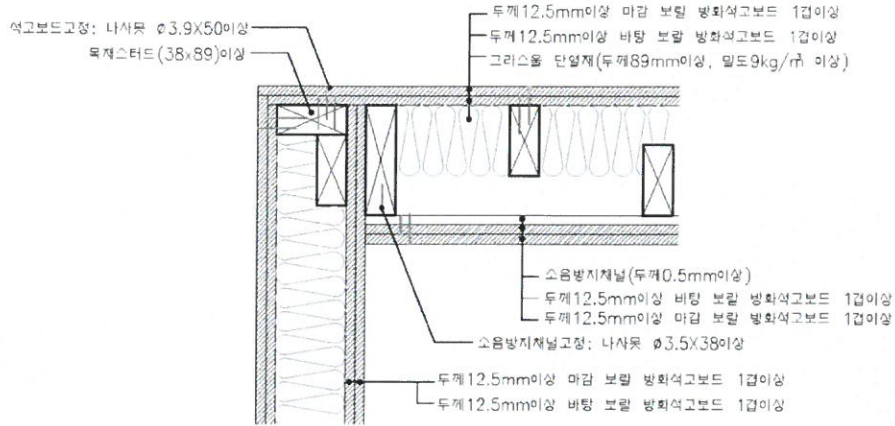
< “ㄱ” 접합 상세도 >
