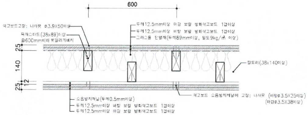
<수평 단면도>
