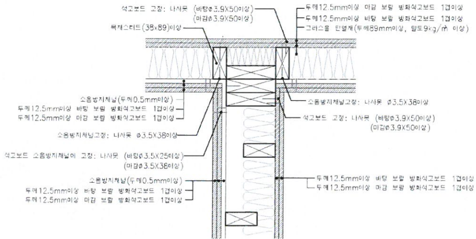
< “T” 접합 상세도 >
