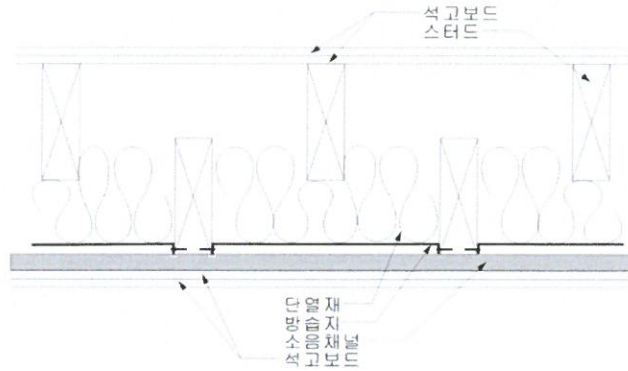
그림 2 단열재의 설치
