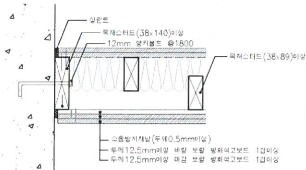
< 벽 접합 상세도 >
