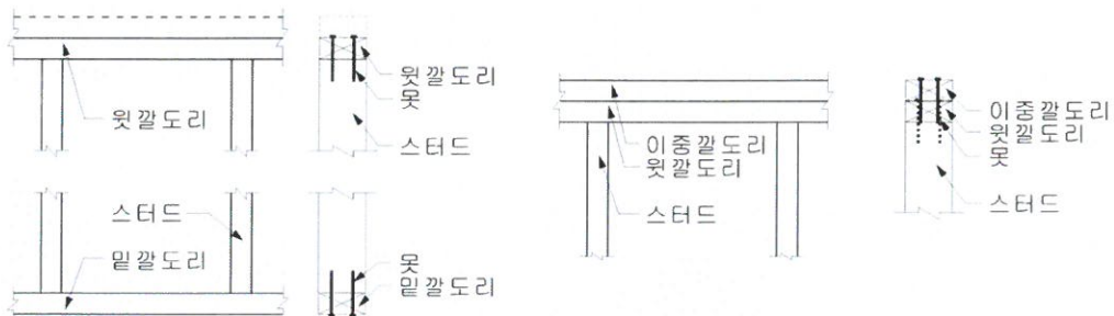
(a) 밑깔도리 및 윗깔도리와 스터드의 고정
