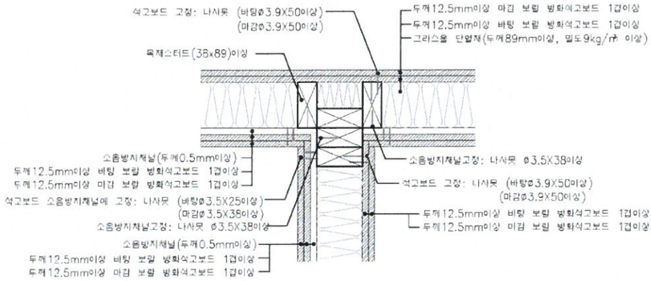
< “T” 접합 상세도 >
