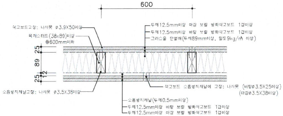
<수평 단면도>
