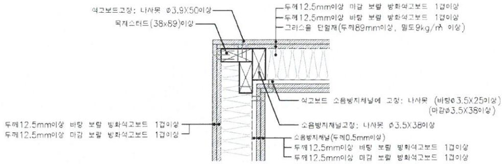
< “ㄱ” 접합 상세도 >
